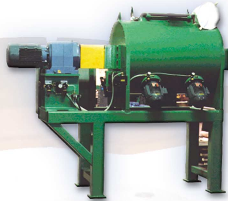
Model M-Series Mezclador de Material 800 ' 3000 Litros de Capacidad
